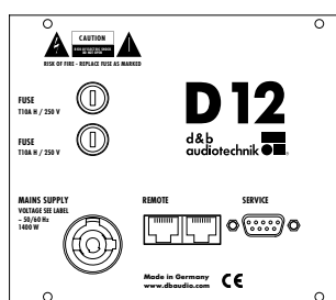
Fig. 27: D12 mains panel
