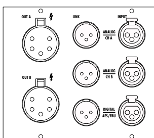
Fig. 28: D12 I/O panel EP5
