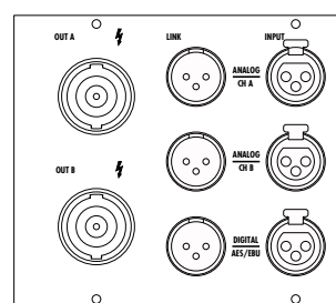
Fig. 30: D12 I/O panel NL4
