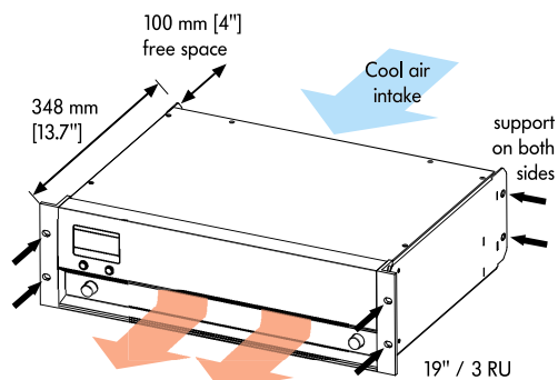
Fig. 21: D12 Installation
