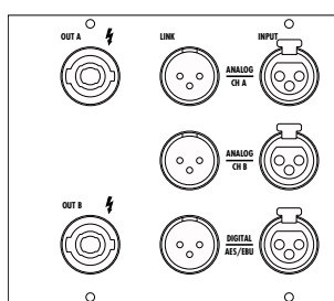
Fig. 29: D12 I/O panel NL4
